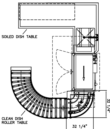
90° Tite turn Unloader
