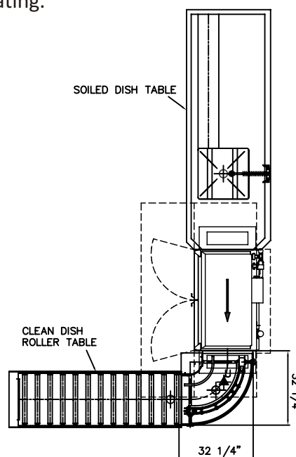
90° Tite turn Unloader
