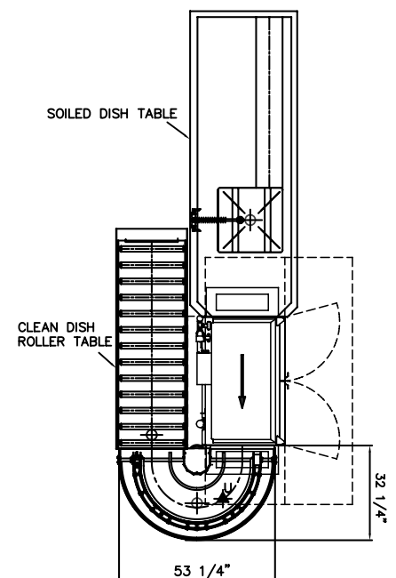
180° Tite turn Unloader
